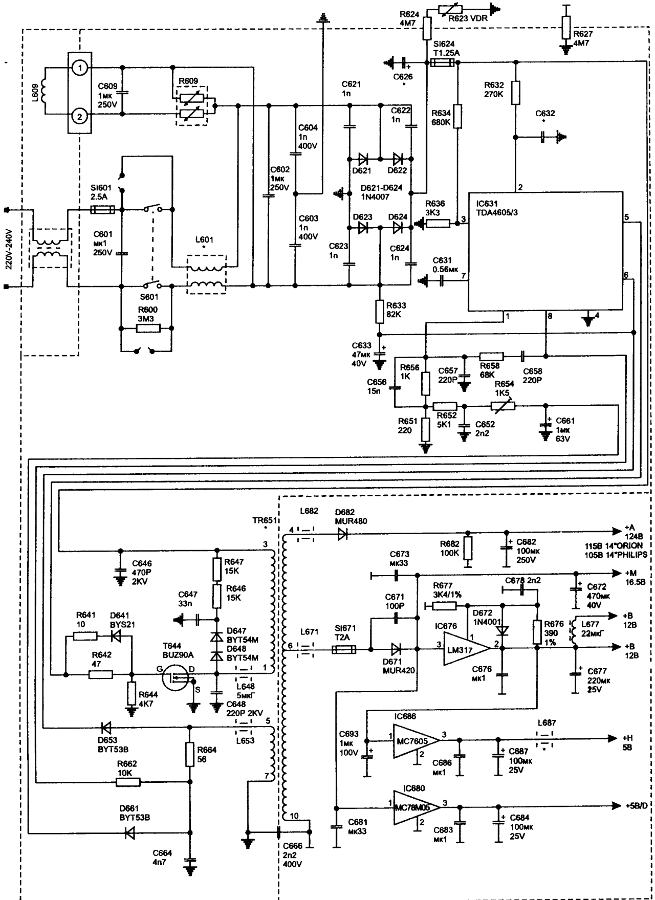
Схема принципиальная источника питания телевизоров «GRUNDIG» CUC6300, P37-060, P40-060, P37-640, P40-640, P42-060, P45-640, 51-060, 51-640, T55-060, T55-640, P50-640
